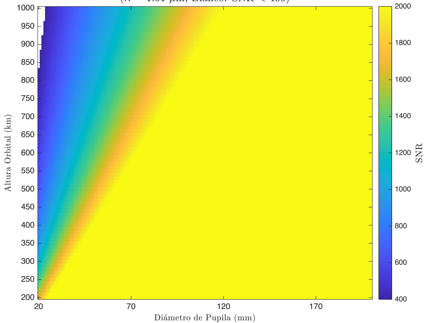
SNR - TMA - Detector 2 ( \lambda = 1.61 \mu\text{m} , Blanco: SNR < 400)
